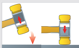
El relleno especial metálico del cabezal evita el retroceso del martillo.
